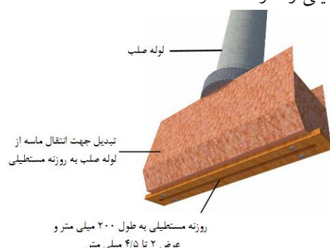
شکل ۴. تبدیل جهت انتقال ماسه از لوله صلب به روزنه مستطیلی
