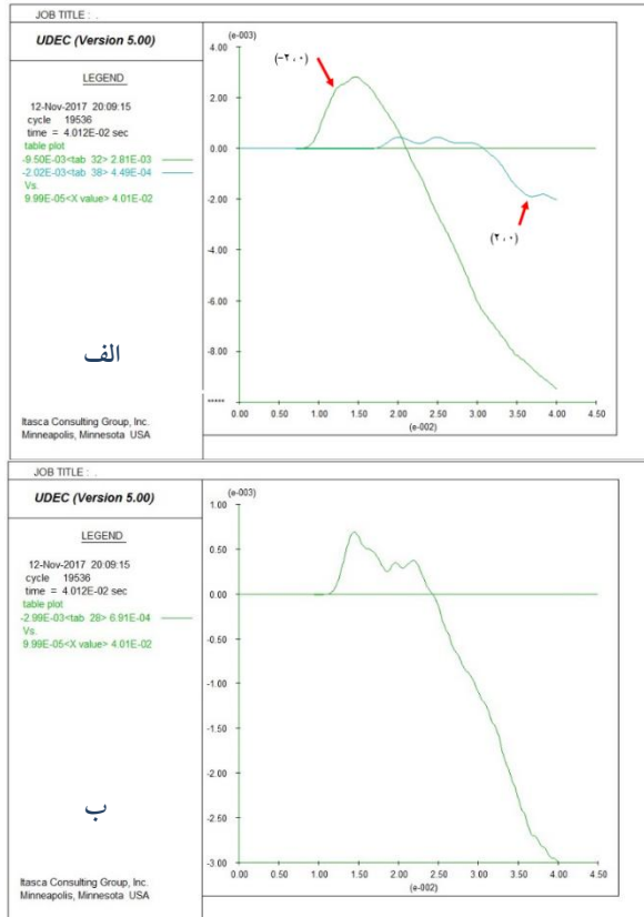
شکل ۱۱. تاریخچهٔ زمانی جابه‌جایی‌های افقی (الف) در نقاط شاهد (۰، ۲-) و (۰، ۲) روی دیوارهٔ سمت چپ و راست رمپ، (ب) در نقطه شاهد (۲/۱، ۰) روی سقف در مدت زمان ۴۰ میلی ثانیه از اعمال بار دینامیکی
