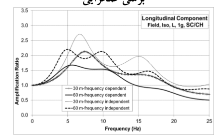
ه) PGA=1g خاک نوع I، مینا سرعت موج برشی صحرائی
