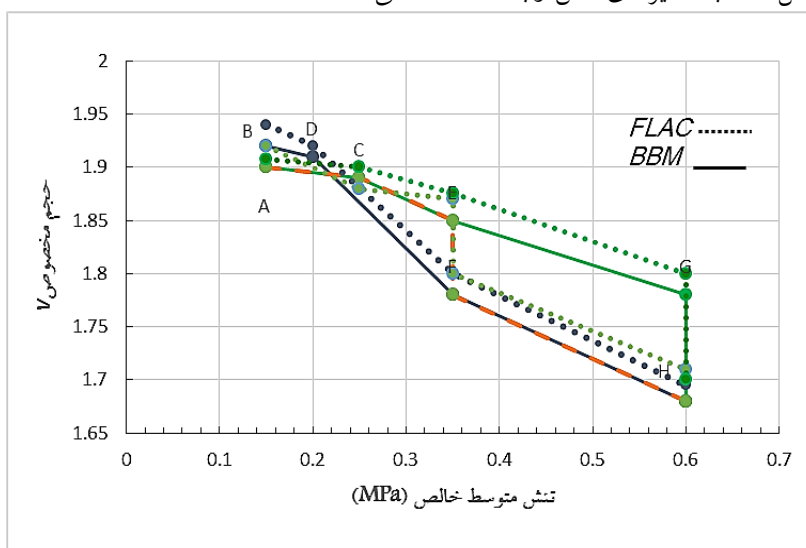
شکل ۵. مقایسه نتایج حاصل از پیاده‌سازی مدل پایه بارسولونا در FLAC و نتایج پژوهش‌های آلونسو (۱۹۹۰).
