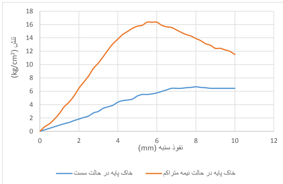
شکل ۸- نمودار تنش - نفوذ سنبه برای خاک پایه در دو حالت سست و نیمه متراکم
