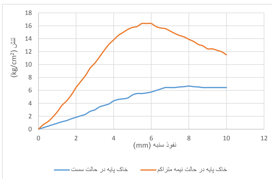
شکل ۸- نمودار تنش - نفوذ سنبه برای خاک پایه در دو حالت سست و نیمه تراکم
