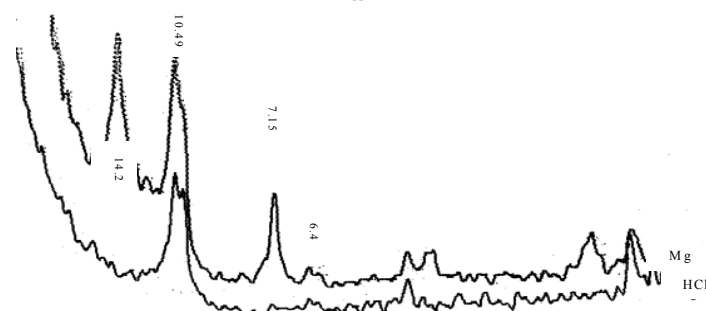
شکل ۵ - دیفراکتوگرام‌های مربوط به پروفیل شماره ۶
