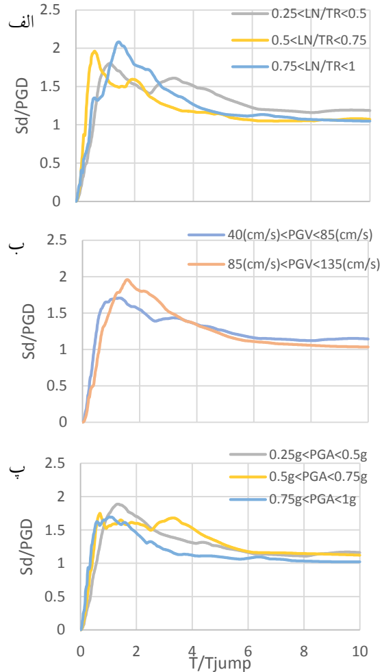
شکل ۷- طیف پاسخ جابجایی نرمال دوسویه با معیار گام پرش زمانی T_{jump} ، (با نماد (BNDS(T_{jump})) )
