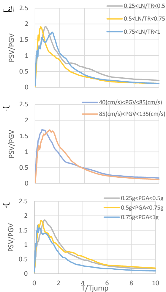
شکل ۸- طیف پاسخ شبه سرعت نرمال دوسویه با معیار گام پرش زمانی T_{jump} ، (با نماد (BNPVS(T_{jump})) )
