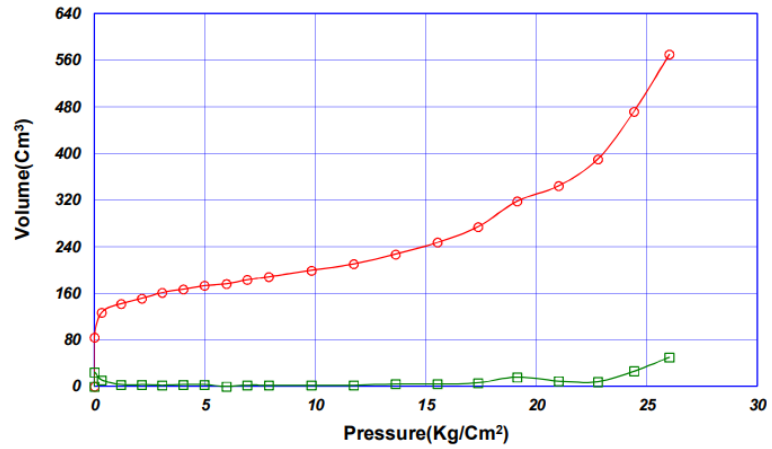
شکل ۱۰. نمونه نتایج آزمایش پرسیمتری که در عمق ۱۵ متری اندازه گرفته شده است. Fig. 10. A sample of pressure test results measured at a depth of 15 meters.
