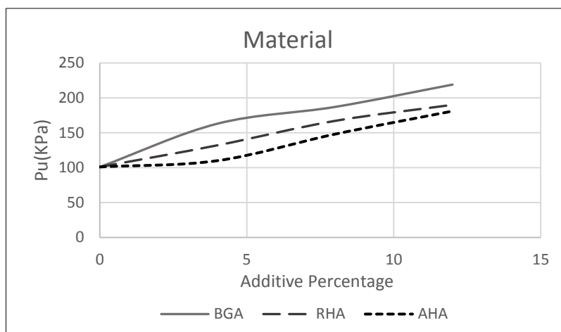
شکل ۵. نمودار مقاومت تک محوری بر حسب درصد افزودنی Fig. 5. Uni-axial strength diagram based on additive percentage
