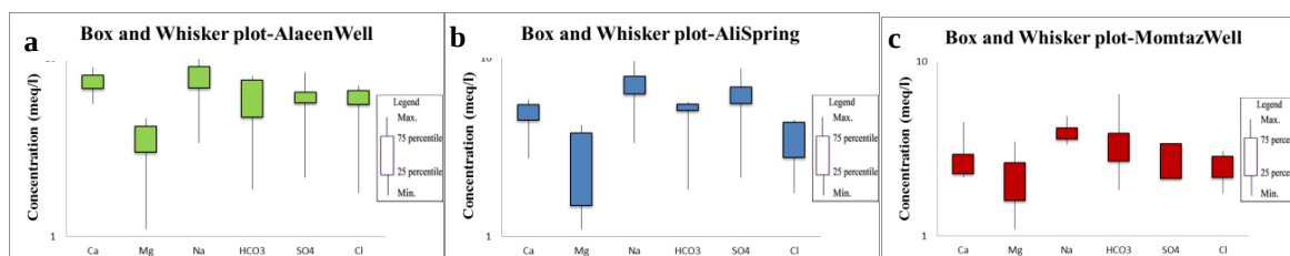
شکل ۲. نمودار جعبه‌ای منابع آبی گستره مطالعاتی شامل: a-چاه علایین، b-چشمه علی شهری و c-چاه ممتاز Fig. 3. Gibbs chart of water resources in the study area, including a) Momtaz well, b) Ali Spring of Shahr-e-Rey, and c) Alaeen well
