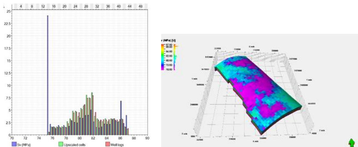
شکل ۱۳. مدل سه بعدی و واریوگرافی تنش مؤثر قائم
