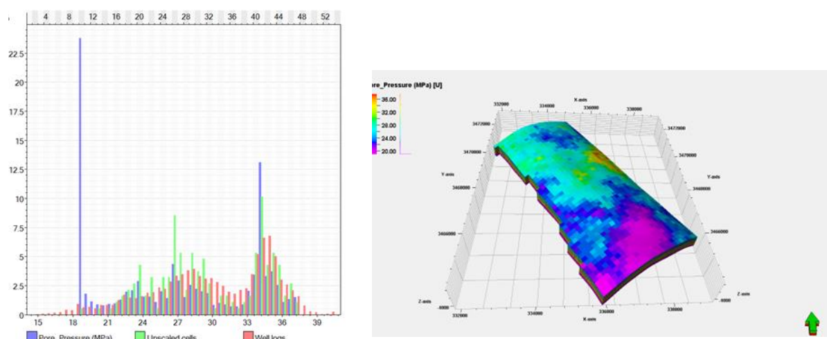
شکل ۱۱. مدل سه بعدی و واریوگرافی فشار منفذی
