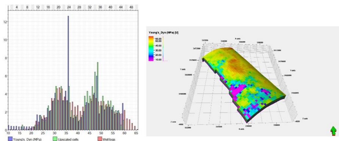
شکل ۵. مدل سه بعدی و واریوگرافی مدول یانگ دینامیکی
