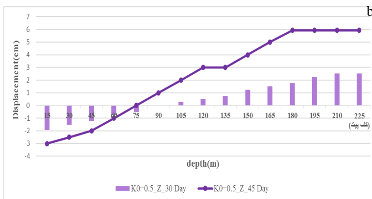
شکل ۶. a. کنتور جابه‌جایی‌ها در راستای Z به صورت سه بعدی بعد از ۳۰ روز برای نسبت تنش افقی به قائم ۰/۵، b. مقدار جابه‌جایی در راستای Z به تفکیک پله بعد از گذر زمان ۳۰ و ۴۵ روز
