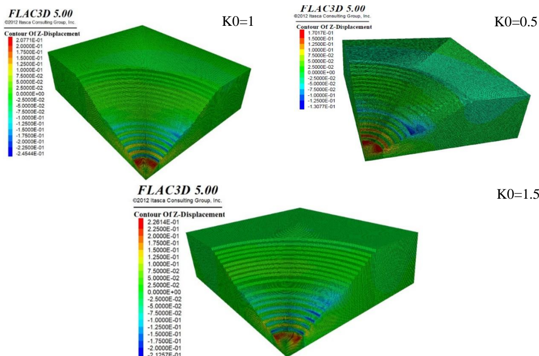
شکل ۸. کنطور جابه‌جایی‌ها در راستای Z در سناریوی سوم برای نسبت‌های تنش افقی به قائم ۱/۵ و ۱، ۰/۵ Fig. 8. Displacement contours in the Z direction in Scenario 3 for horizontal-to-vertical stress ratios of 0.5, 1, and 1.5
