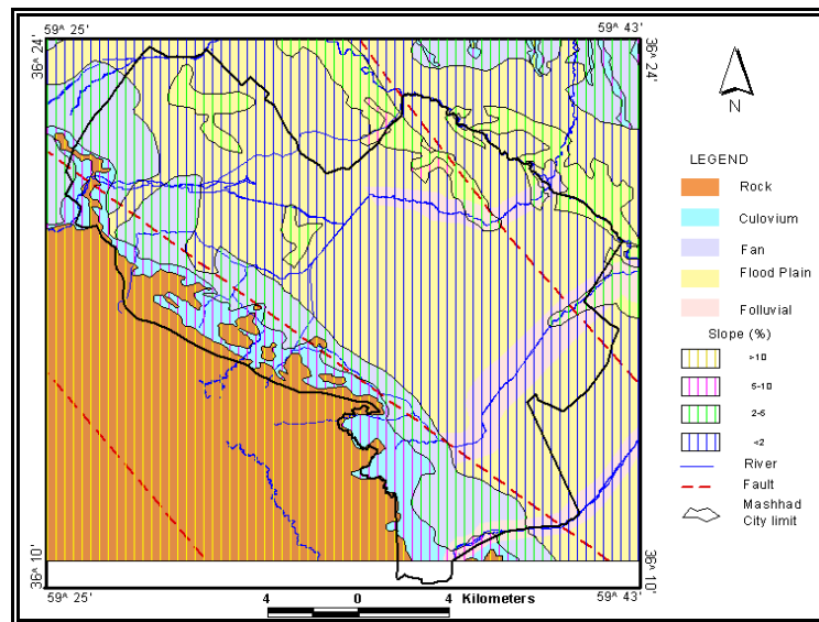
شکل ۲. نقشه پهنبندی شهر مشهد از نظر محیط رسوبی (حافظی مقدس ۱۳۸۶)
