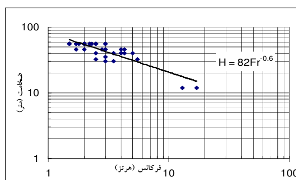
شکل ۸. رابطهٔ بین ضخامت و فرکانس آبرفت
