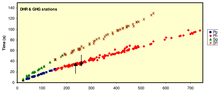
شکل ۱۲. نمودار زمان-مسافت موج‌های P و S به روش دوا ایستگاهی در امتداد مسیرهای دهرش و قلغزی شکل ۱
