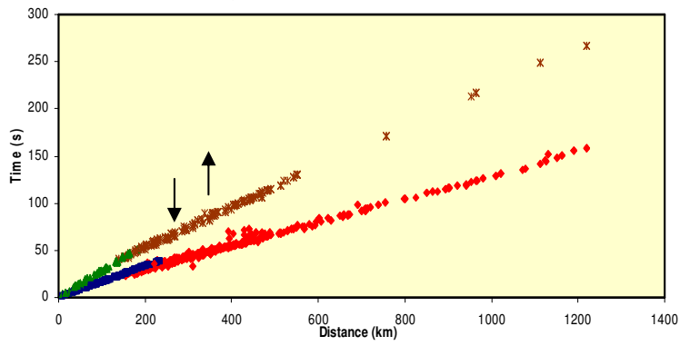
شکل ۱۷. نمودارهای زمان-مسافت موج‌های P و S در امتداد همه مسیرهای شکل ۱
