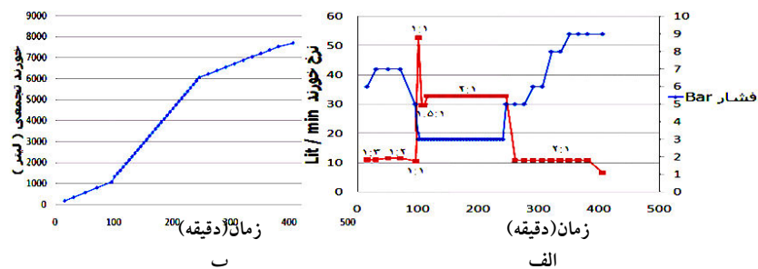
شکل ۸ الف) نمودار نرخ خوردن- زمان - فشار مقطع ۵۰-۴۰ از گمانه (PR29) ب) نمودار خوردن تجمعی- زمان مقطع ۵۰-۴۰ از گمانه (PR29)
