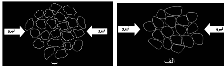
شکل ۱۳. تأثیر قفل و بست سنگ‌دانه‌ها در افزایش مقاومت فشاری بتن (الف- گرانیت ب- لوماشل، دولومیت)
