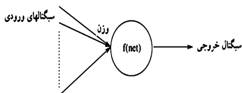
شکل ۱. نرون مصنوعی [۲۸]
