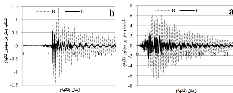
شکل ۵. تاریخچه زمانی شتاب رسیده به سطح زمین برای عمق سنگ‌بستر برابر با ۱۰ متر در اثر
