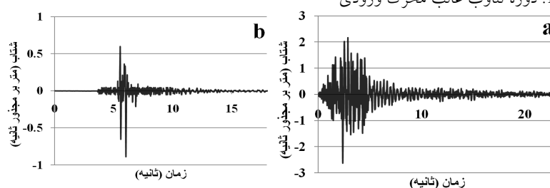
شکل ۲. تاریخچه زمانی محرک های ورودی قوی (a) و ضعیف (b)
