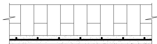
شکل ۴. مقطع میان‌قاب حایل بنایی تقویت شده
