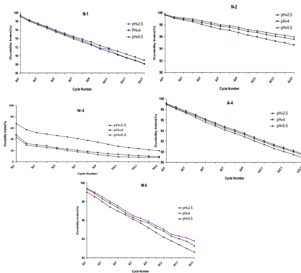
شکل ۵. نتایج آزمایش دوام و ارتفتگی بر روی نمونه‌های بررسی شده با استفاده از محلول‌های با اسیدیته مختلف (علائم موجود در شکل، در جدول ۱ توصیف شده‌اند).
