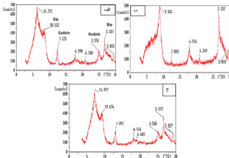
شکل ۳. طیف انکسار اشعه X در نمونه A 18 (الف) در سه حالت (الف) نمونه خشک شده در دمای طبیعی، (ب) نمونه حرارت داده شده (ج) نمونه عمل آوری شده با اتیلن گلاکول نشان می‌دهد، چنان‌که ذکر شد کانی‌های رسی موجود در سنگ‌های مارنی ساختگاه سد از نوع ایلیت و کائولینیت هستند.
