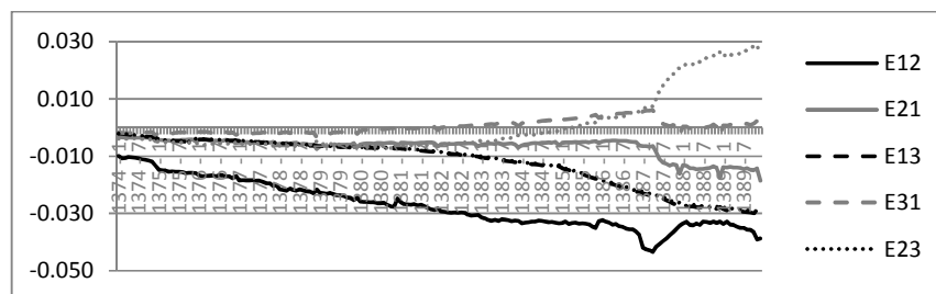
نمودار ۳. روند کشش قیمتی متقاطع مولفه های پولی با استفاده از مدل EASI
