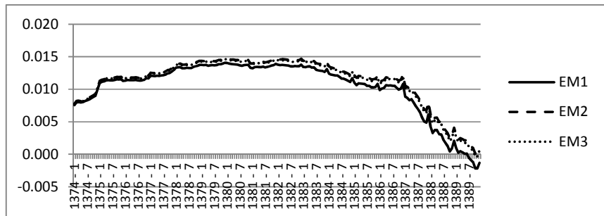
نمودار ۱. روند کسش درآمدي مولفه‌های پولی با استفاده از مدل EASI
