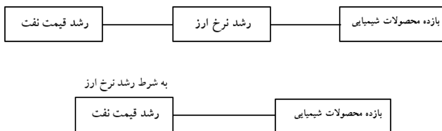
شکل ۳: ساختار D-vine
