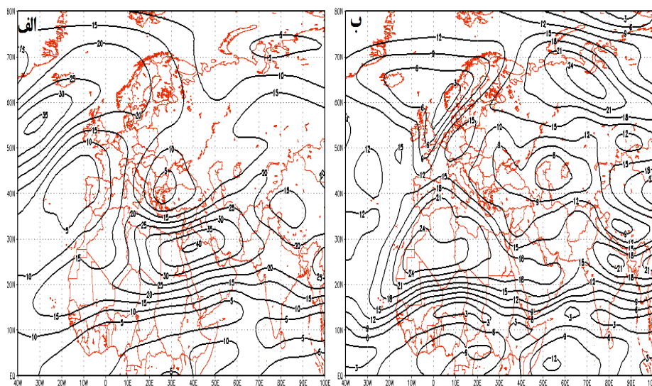
شکل (۱۱) الگوی شدت باد تراز ۴۰۰ هکتوپاسکال برای ردیابی رودباد الف: فاز مثبت دسامبر ۱۹۹۱، ب: فاز منفی آوریل ۱۹۸۶
