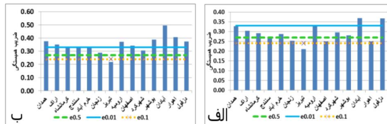
شکل (۱۰). مقادیر همبستگی ناهنجاری بارش هر ایستگاه با تغییرات ارتفاع تراز ۳۰۰ (الف)، دما تراز ۴۰۰ (ب). دریا در منطقه غرب دریای مدیترانه (ب).
