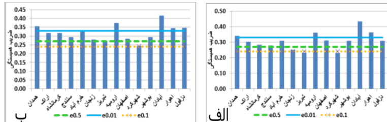
شکل (۱۱). مقادیر همبستگی ناهنجاری بارش هر ایستگاه با تغییرات دما تراز ۹۲۵ (الف)، دما تراز ۸۵۰ (ب). هکتوپاسکال در منطقه غرب دریای مدیترانه (ب).
