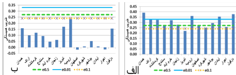
شکل (۱۲). مقادیر همبستگی ناهنجاری بارش هر ایستگاه با تغییرات دما تراز ۵۰۰ (الف)، دما تراز ۳۰۰ (ب). هکتوپاسکال در منطقه غرب دریای مدیترانه (ب).
