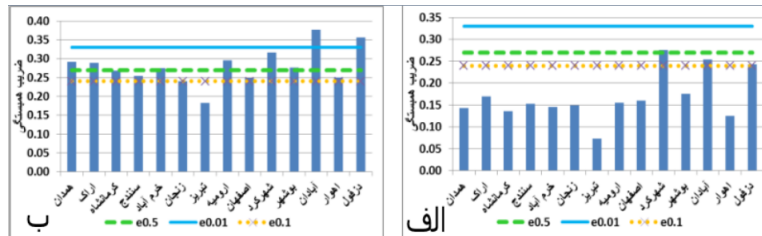
شکل (۹). مقادیر همبستگی ناهنجاری بارش هر ایستگاه با تغییرات ارتفاع تراز ۸۵۰ (الف)، ارتفاع تراز ۳۰۰ (ب). مقادیر همبستگی ناهنجاری بارش هر ایستگاه با تغییرات ارتفاع تراز ۸۵۰ (الف)، ارتفاع تراز ۳۰۰ (ب). مقادیر همبستگی ناهنجاری بارش هر ایستگاه با تغییرات ارتفاع تراز ۸۵۰ (الف)، ارتفاع تراز ۳۰۰ (ب). مقادیر همبستگی ناهنجاری بارش هر ایستگاه با تغییرات ارتفاع تراز ۸۵۰ (الف)، ارتفاع تراز ۳۰۰ (ب).
