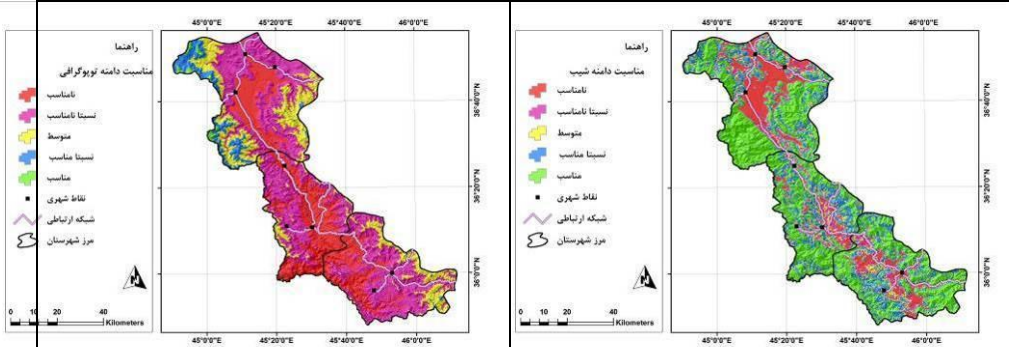
شکل (۲). نقشه شیب حوضه آبریز زاب
