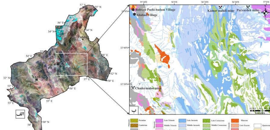
شکل (۱). (الف) موقعیت منطقه مورد مطالعه بر روی تصویر ماهواره ای TM استان یزد و (ب) نقشه زمین شناسی منطقه مورد مطالعه بر گرفته از نقشه ۱/۲۵۰۰۰۰ آبدوخی (آقناباتی و سعیدی، ۱۳۹۰).
