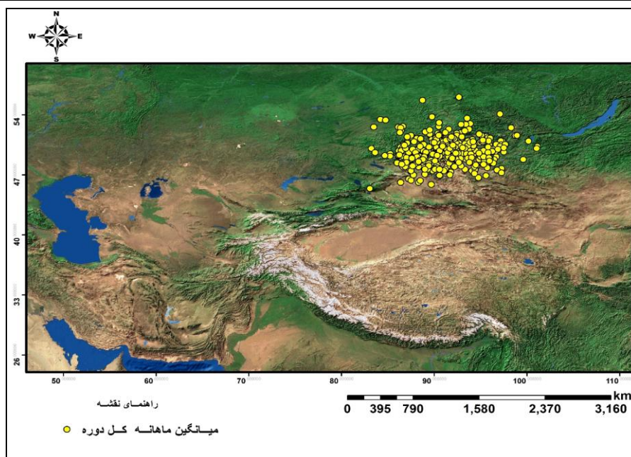
شکل (۱). منطقه مورد مطالعه و محدوده تشکیل هسته پرفشار سبیری
