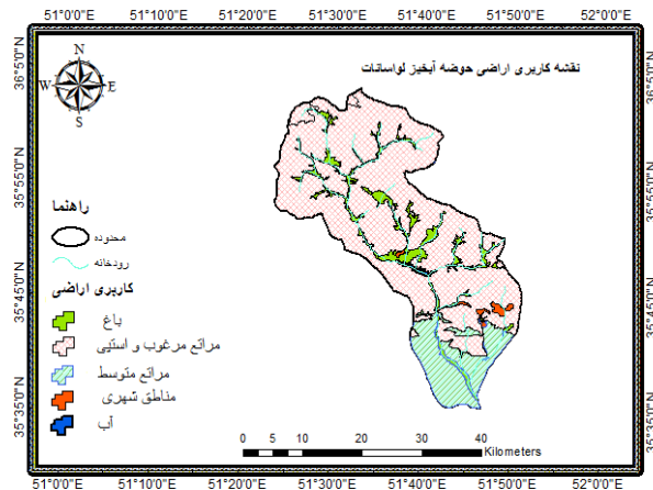
شکل (۹). نقشه کاربری اراضی حوضه آبخیز لواسانات
