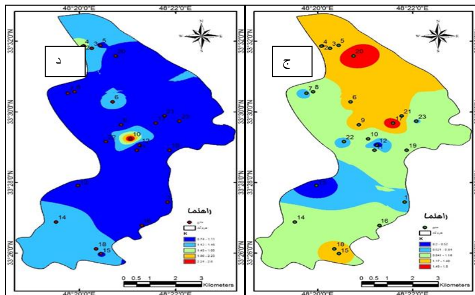
شکل (۴). تغییرات میزان (k) در چاههای شرب خرم آباد (الف) در فصل بهار (ب) در فصل تابستان (ج) در فصل پاییز (د) در فصل زمستان
