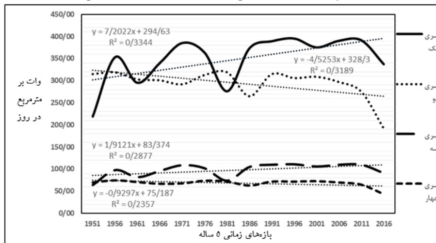
شکل (۴). سری یک- بیش‌ترین تغییرات افزایشی تابش ورودی به سطح زمین در شمال استان سیستان و بلوچستان، سری دو- بیش‌ترین تغییرات کاهش‌ی تابش ورودی به سطح زمین در شمال استان فارس، سری سه- بیش‌ترین تغییرات افزایشی تابش خروجی از سطح زمین در شمال استان سیستان و بلوچستان، سری چهار- بیش‌ترین تغییرات کاهش‌ی تابش خروجی از سطح زمین در شمال استان فارس، در ماه می
