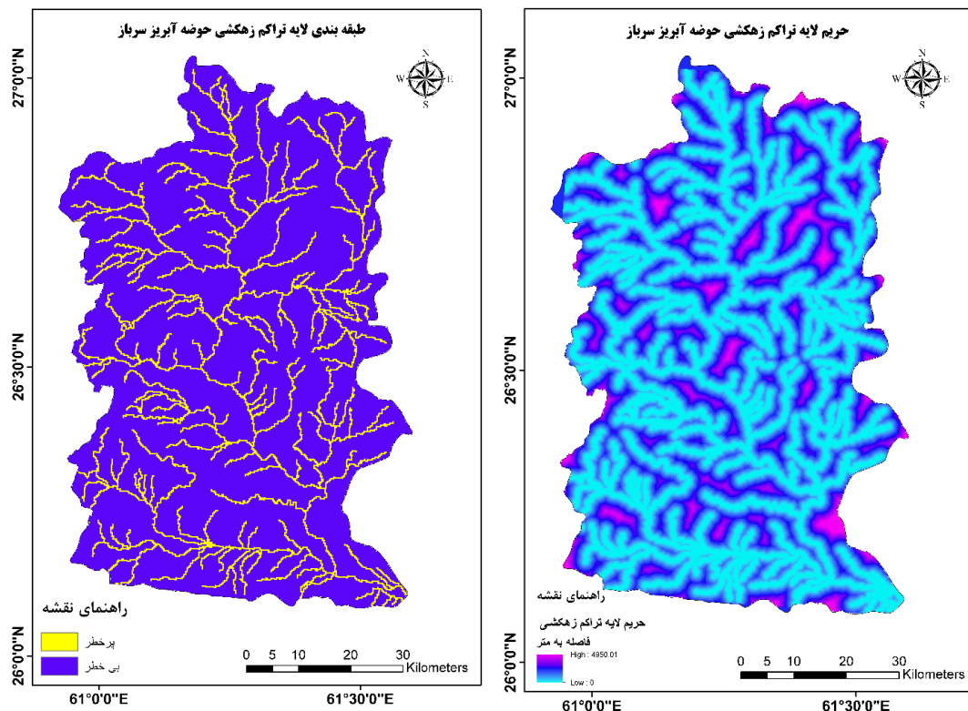
شکل (۱۶). طبقه‌بندی لایه تراکم زهکشی از نظر پتانسیل سیل خیزی (منبع: نگارندگان)
