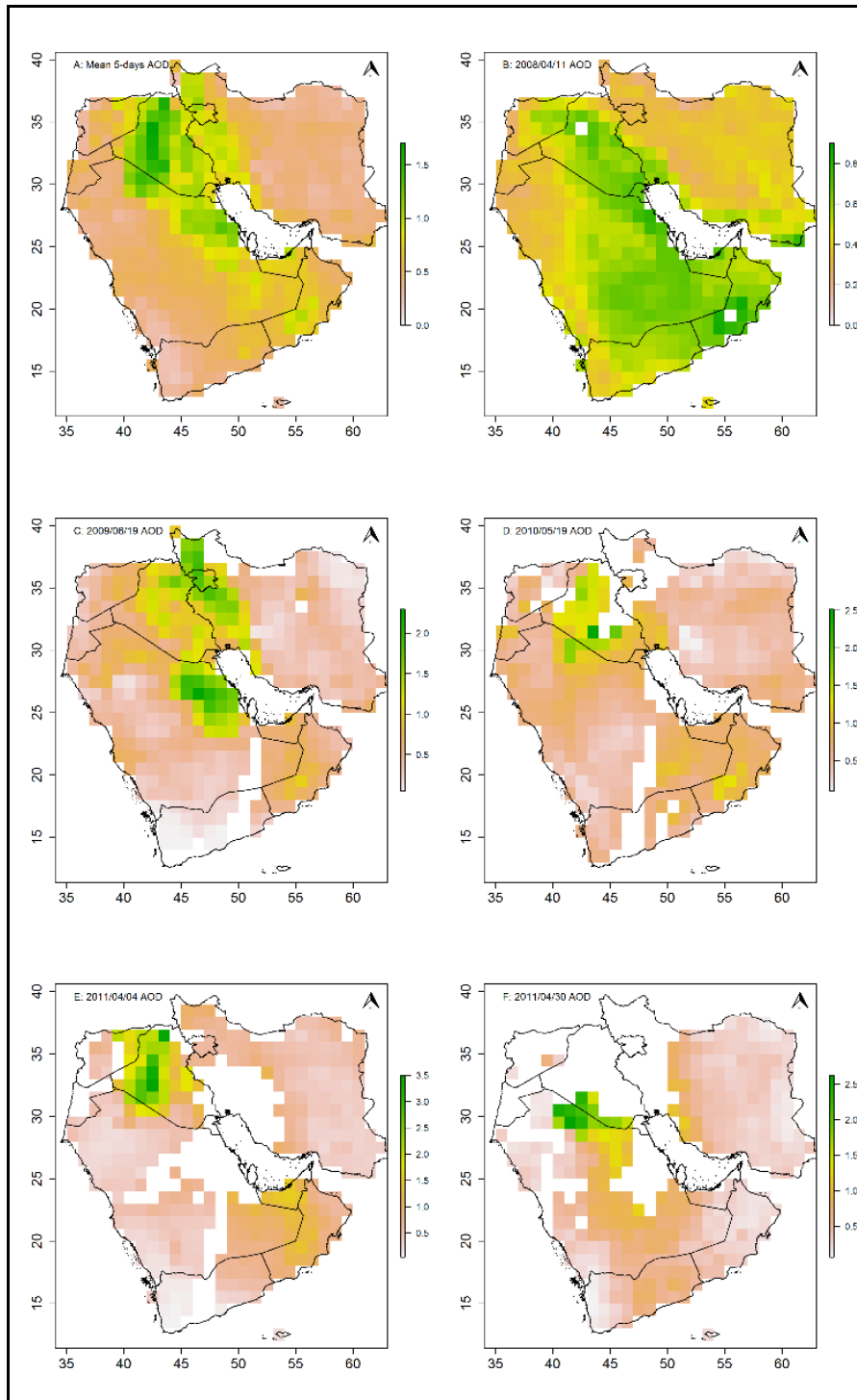
شکل (۱۰). پراکنش مکانی عمق نوری آئروسول MODIS (AOD 550nm) بر روی خاورمیانه، A: میانگین ۵-روزه فرین‌های گردوغبار، B: فرین ۲۰۰۸/۰۴/۱۱، C: ۲۰۰۹/۰۶/۱۹، D: ۲۰۱۰/۰۵/۱۹، E: ۲۰۱۱/۰۴/۰۴ و F: ۲۰۱۱/۰۴/۳۰
