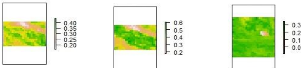
نمودار پیکسلی مربوط به سال ۲۰۰۰ نمودار پیکسلی مربوط به سال ۲۰۰۴ نمودار پیکسلی مربوط به سال ۲۰۰۹
