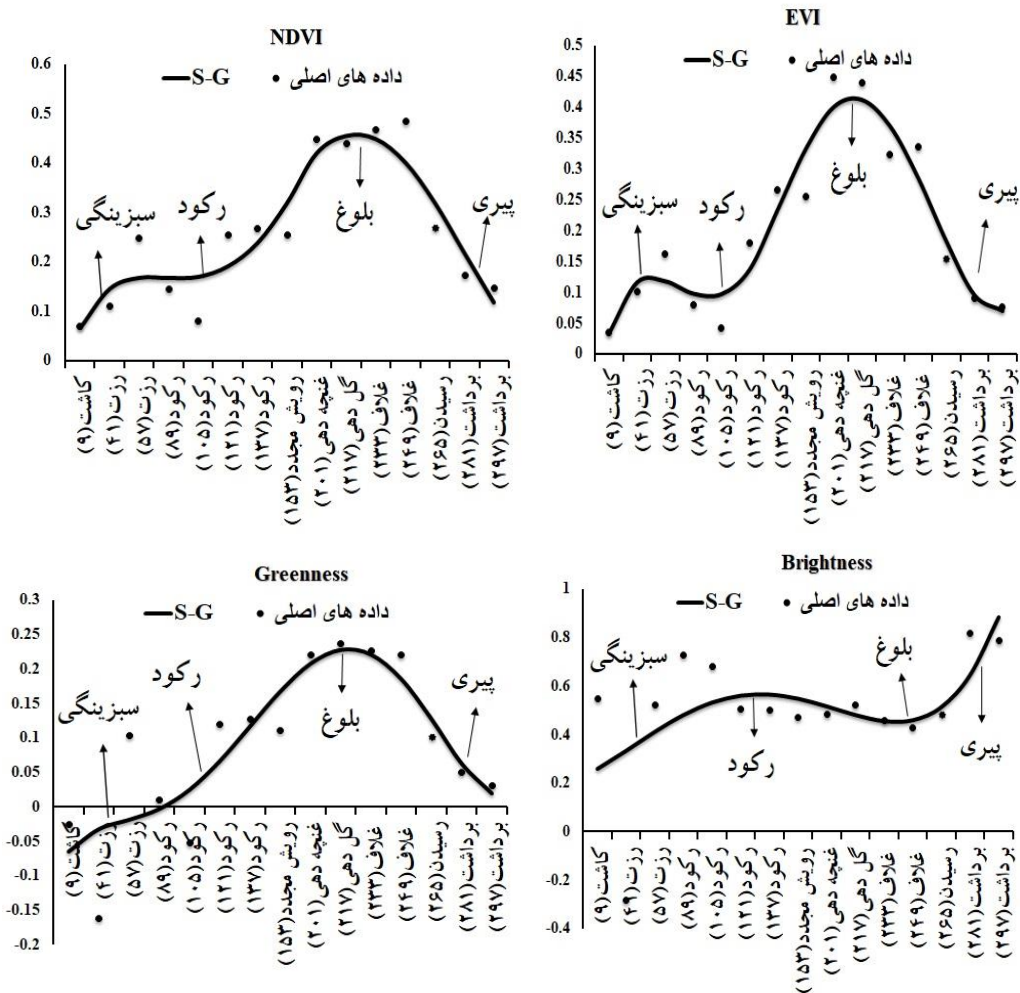
شکل (۳). منحنی هموار شده شاخص های گیاهی سنجش از دور توسط مدل S-G و مراحل اصلی فنولوژی سنجش از دور کلزا (محور افقی شامل مراحل فنولوژی دیده بان شده و اعداد داخل پیرانتز نشان دهنده تعداد روز بعد از مرحله کاشت می باشد)
