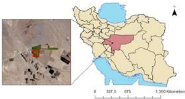
شکل (۱). منطقه مورد مطالعه به همراه تصویر RGB (ادغام سه باند قرمز، سبز و آبی برای تولید تصویر رنگی) سنجنده OLI ماهواره لندست ۸ از مزرعه - منبع: نگارندگان
