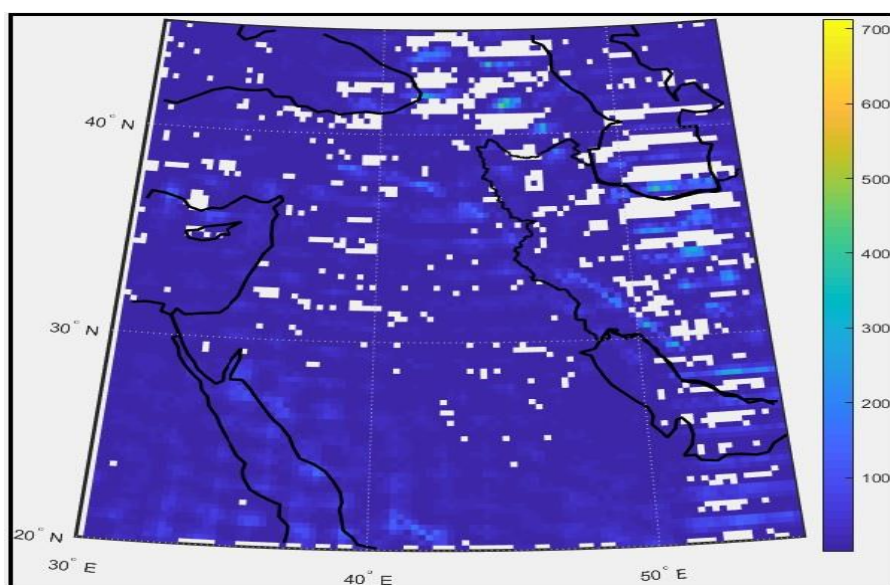
شکل (۹). مکان چرخندزایی و گذر چرخندی در ماه ژانویه در طول سال‌های آماری ۱۹۷۹-۲۰۱۶ (آبی پررنگ چرخندزایی ضعیف و طیف رنگی متماثل به زرد چرخندزایی، مربع‌های سفید نشانه عدم رخ داد چرخندزایی)
