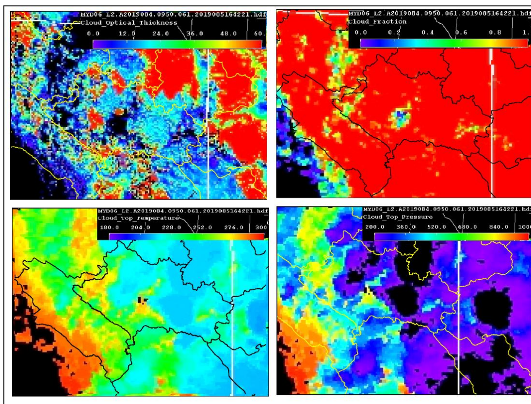
شکل (۶). فاکتورهای میکروفیزیکی ابرهای مولد رخداد بارش ۲۵ مارس ۲۰۱۹ (۵ فروردین ۱۳۹۸) مستخرج از محصول ابر سنجنده MODIS
