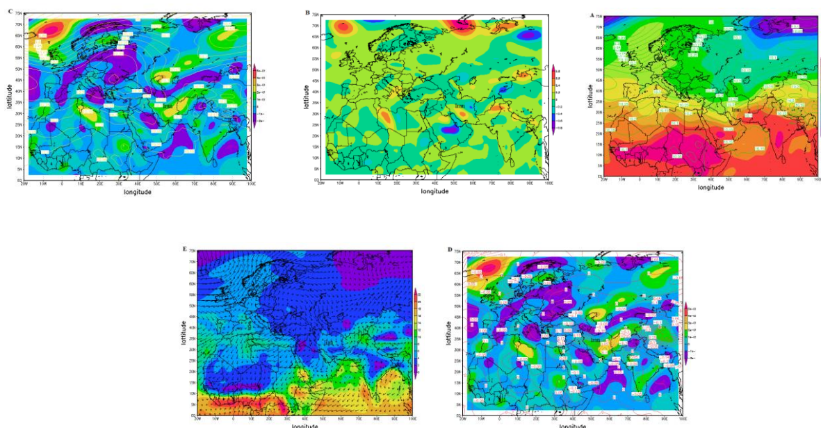
شکل (۸). (A): دما (سلسیوس، °C) و فشار (هکتوپاسکال، hpa) تراز دریا؛ (B): جبهه تراز دریا (کلون بر متر بر ثانیه 10^{-1} \text{ Pa s}^{-1} )؛ (C): تاوایی (متر بر ثانیه 10^{-1} \text{ Pa s}^{-1} ) و فشار تراز دریا (هکتوپاسکال، hpa) (D): تاوایی (متر بر ثانیه 10^{-1} \text{ Pa s}^{-1} ) و امگا (پاسکال بر ثانیه 10^{-1} \text{ Pa s}^{-1} ) تراز دریا (E): باد مداری و نصف‌النهاری و شار همگرایی رطوبت (گرم بر کیلوگرم 10^{-1} \text{ Pa s}^{-1} ) تراز دریا.
