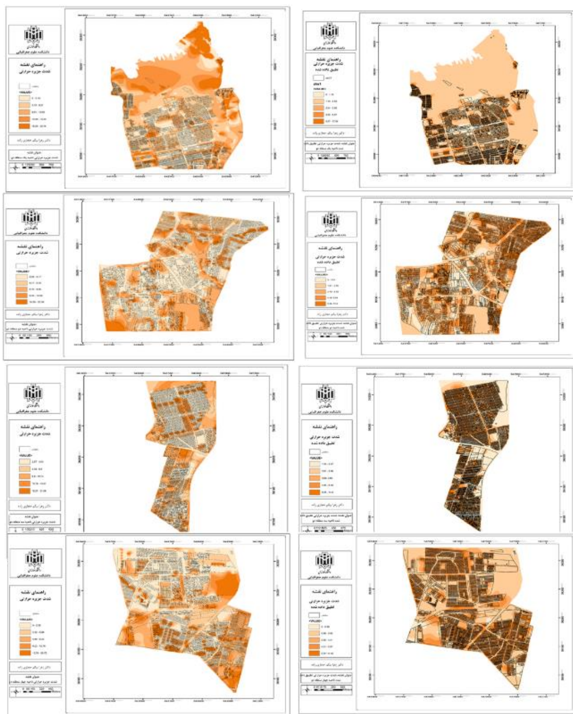
شکل (۸). نقشه حداکثر شدت جزیره حرارتی ناحیه (۱-۴) (سمت چپ از بالا به پایین) و حداکثر شدت جزیره حرارتی تطبیق داده شده ناحیه (۴-۱) منطقه دو تهران (سمت راست از بالا به پایین)
