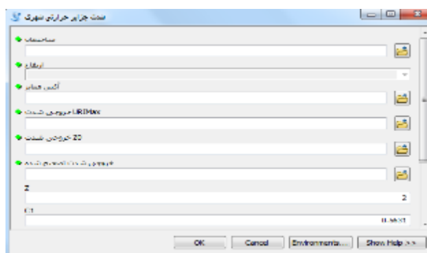
شکل (۴). پنجره ورودی برنامه THIS جهت شبیه‌سازی حداکثر شدت جزیره حرارتی
