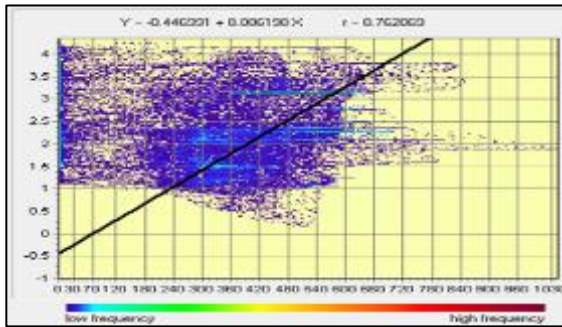
شکل (۲۰). تراکم ساختن و سرعت باد در مناطق سه‌گانه
