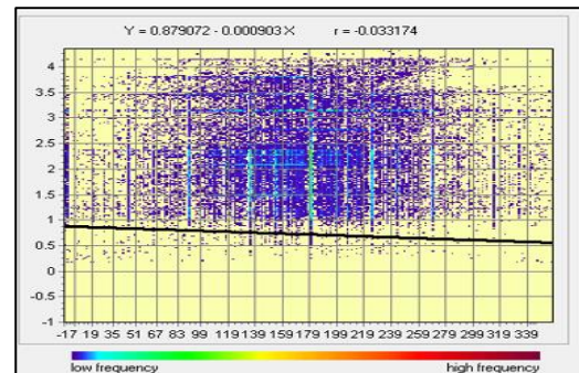
شکل (۲۱). جهت و سرعت باد در مناطق سه‌گانه
