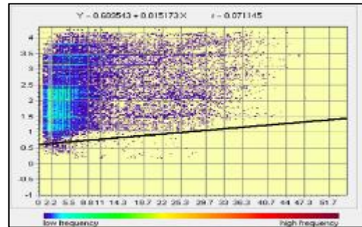
شکل (۱۹). شیب و سرعت باد در مناطق سه‌گانه
