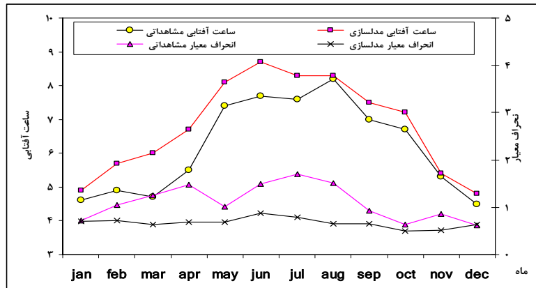
شکل (۱) نمودار میانگین های ماهانه مشاهداتی و شبیه سازی شده ساعت آفتابی و همچنین انحراف معیار آنها در ایستگاه گرگان (۲۰۰۷-۱۹۹۳)
