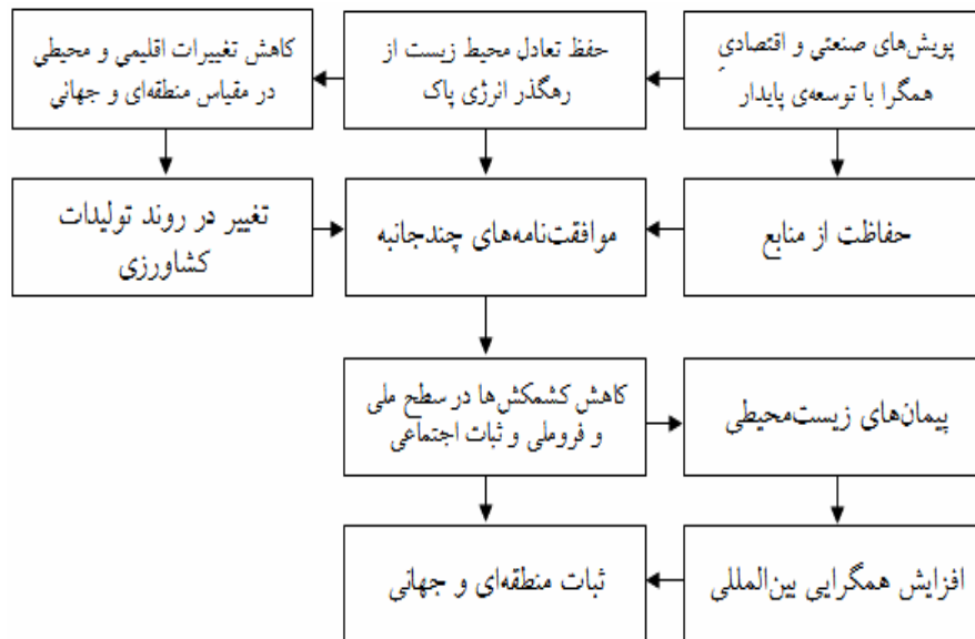
شکل (۴) نمودار تأثیر فرسای محیط بر کشمکش‌های جهانی (ترسیم از نگارنده)
