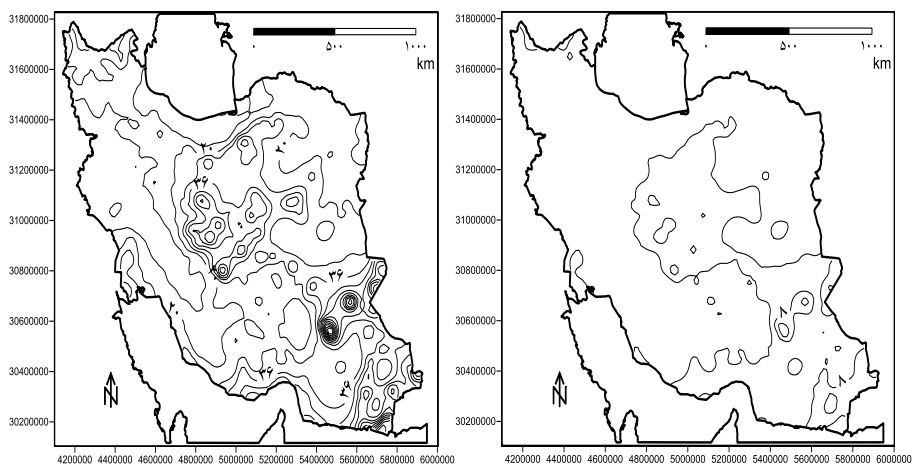
شکل ۸) دوره‌ی بازگشت دو روزه‌ی بارش زمستان (شکل ۹) دوره‌ی بازگشت سه روزه‌ی بارش زمستان
