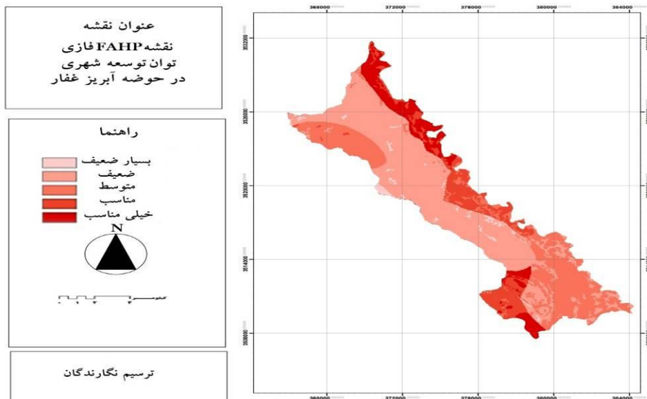
شکل (۹) نقشه نهایی ارزیابی توان توسعه شهری در حوضه آبریز غفار با استفاده از FAHP فازي (مأخذ: محاسبات و ترسیم نگارندگان، ۱۳۹۲)
