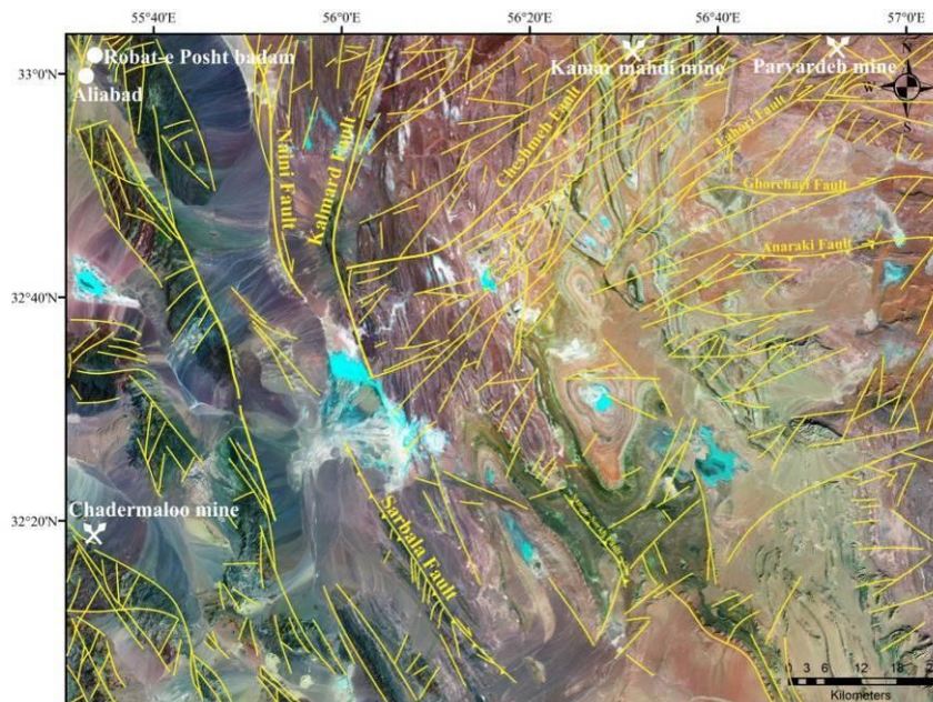
شکل (۲). الگوی گسل ها در منطقه مورد مطالعه بر روی تصویر ماهواره ای (TM) ماخذ: http://glcfapp.glcg.umd.edu:8080/esdi/index.jsp
