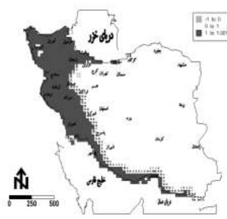
شکل (۹). روند دمای ماه زولای در قلمرو ایران طی دوره آماری ۲۰۱۵-۲۰۵۰
