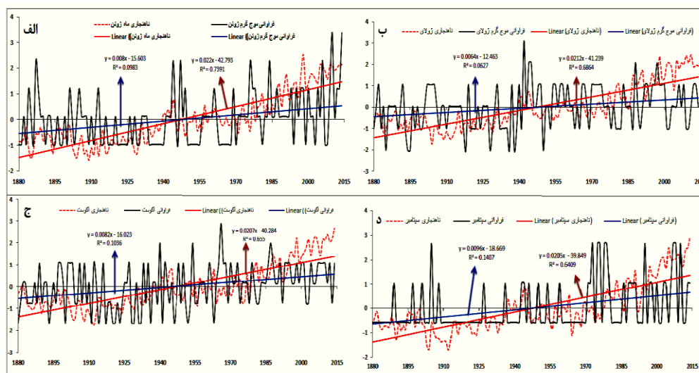
شکل (۹). نمودار مقایسه‌ای و استاندارد شده‌ی ماهانه‌ی فراوانی وقوع امواج گرمایی با ناهنجاری دمایی اقیانوس و خشکی در منطقه شمال‌غرب ایران، الف (ژوئن)، ب (ژولای)، ج (آگوست)، د (سپتامبر) از سال ۱۸۸۰ تا ۲۰۱۴.
