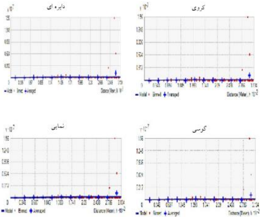
شکل (۷): نیم پراش نگار (دایره ای، کروی، نمایی و گوسی) تجاری در مدل کریجینگ معمولی.
